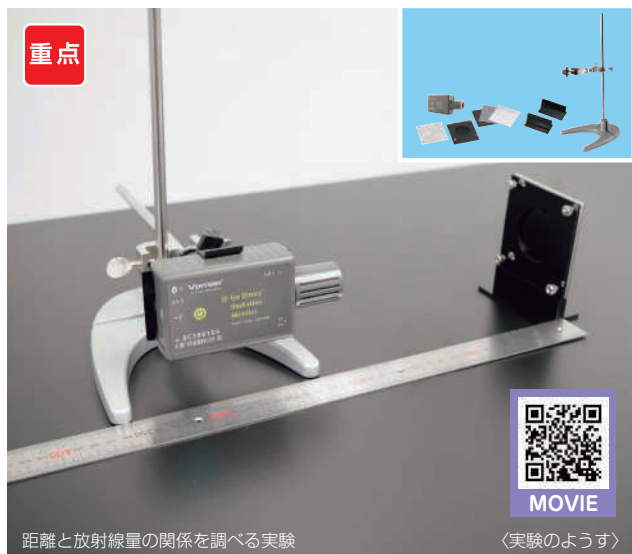
距離と放射線量の関係を調べる実験
